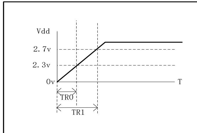
图 8-1 上电复位时间示意图
