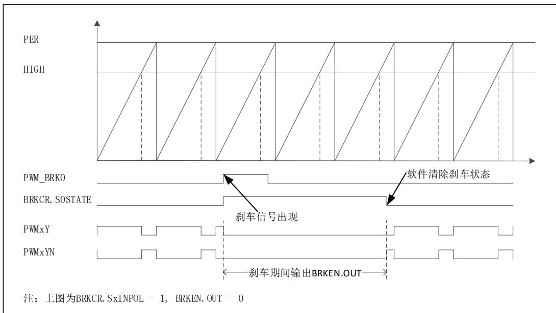
图 6-63 刹车示意图
