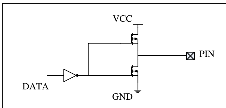
图 6-8 推挽输出
