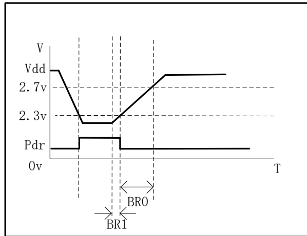
掉电复位示意图
