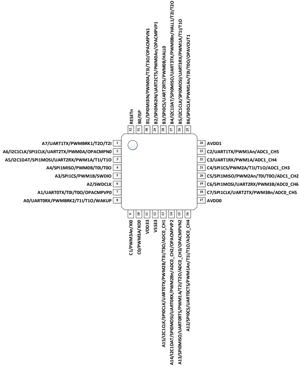
图 5-3 KBT7 封装管脚配置图
