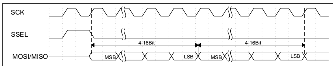
图 6-44 SSI 模式连续输出波形
