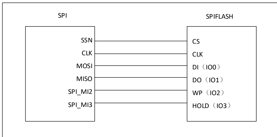
图 6-53 SPIFLASH 四线模式外部连接图
