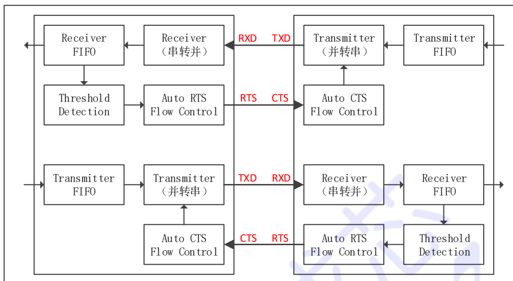
图 6-23 硬件流控
