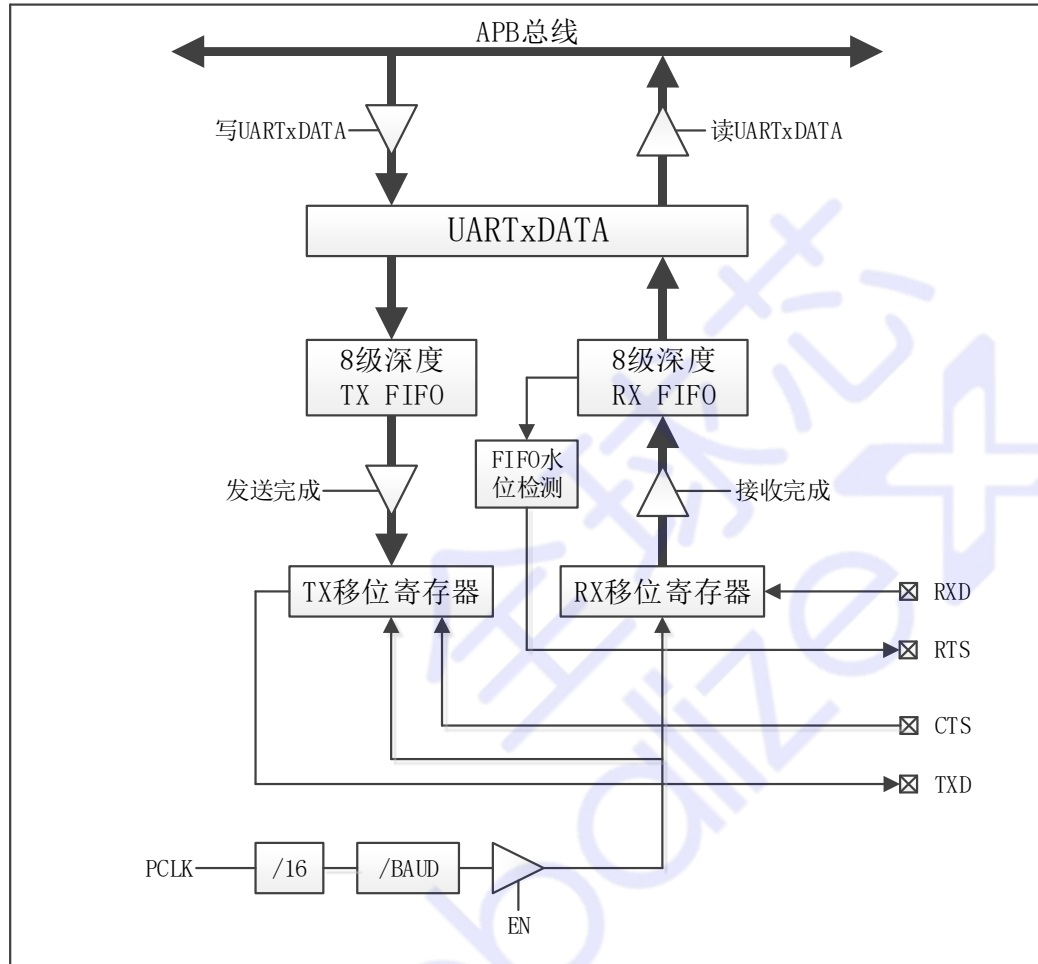
图 6-17 UART 结构图
