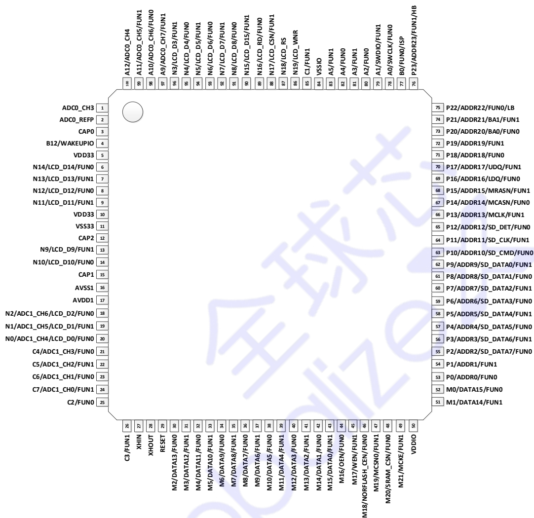
图 5-3 SWM320VET7 封装管脚配置
