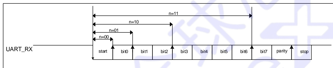
图 6-19 AUTOBAUDBITS 配置图
