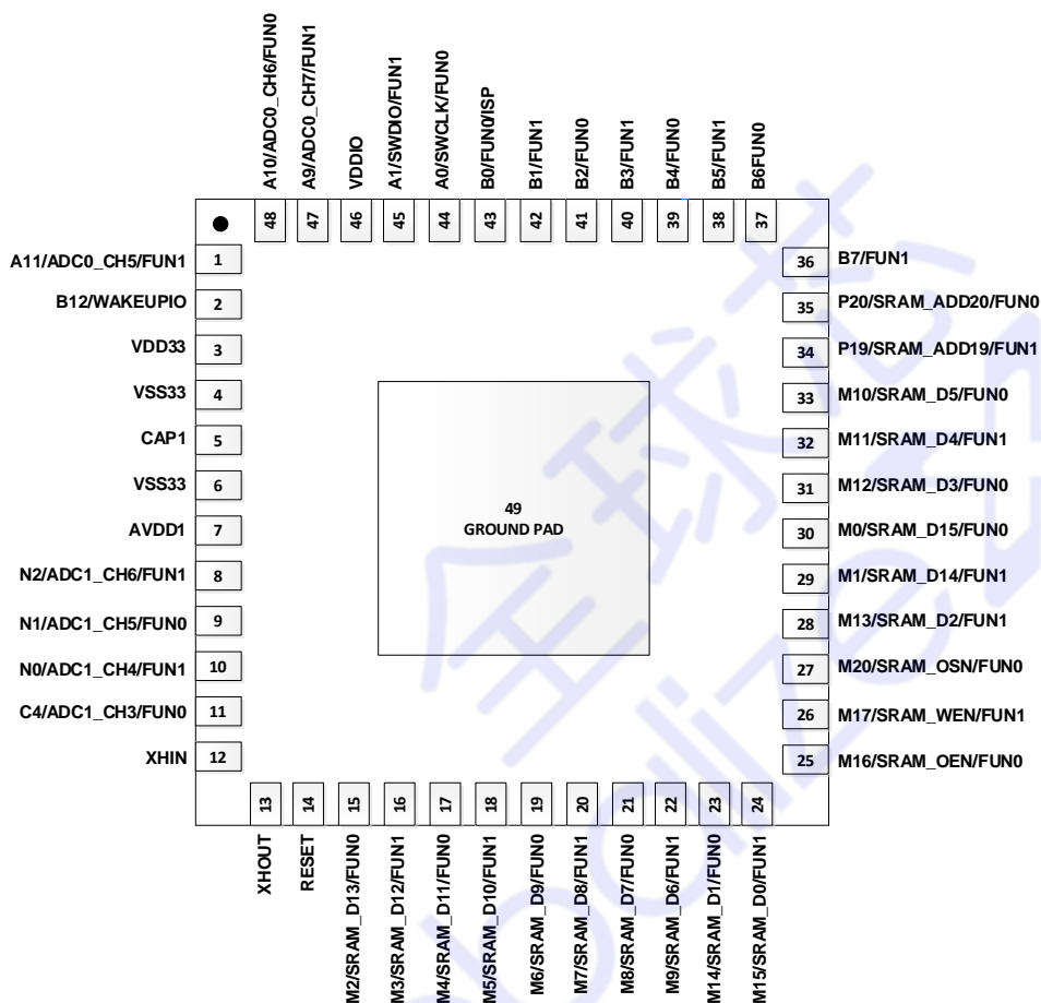
图 5-1 SWM320CEU7 封装管脚配置
